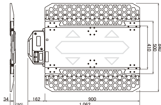
ZAK-06W-10 パッド外観図
